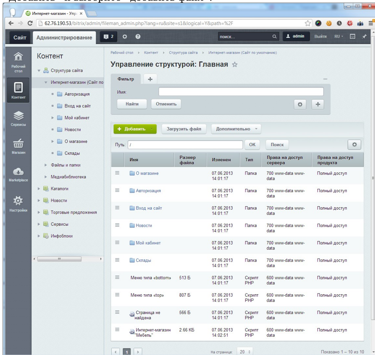
Рисунок 6. Добавление страницы.
